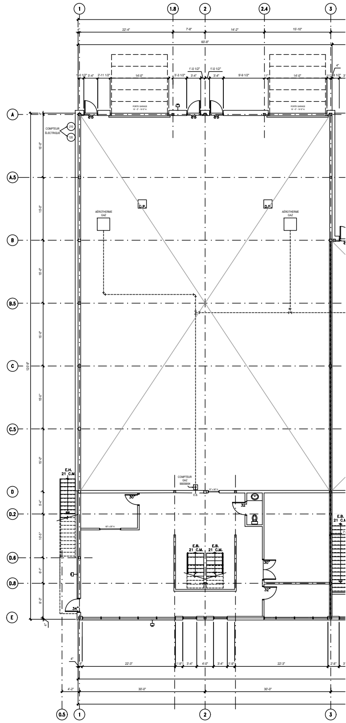
ÉTAGE - SUITE 150
